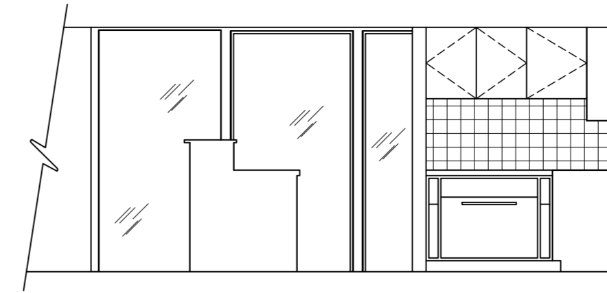
4 S. ELEVATION KITCHEN
