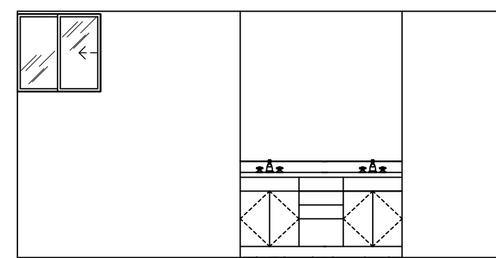
2 N. ELEVATION BEDROOM 1
