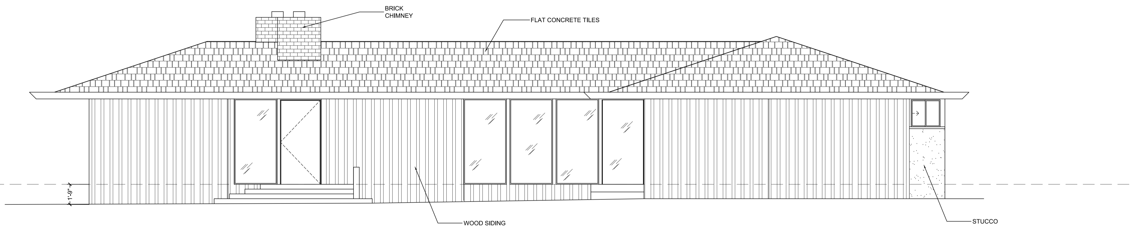
2 N. ELEVATION
