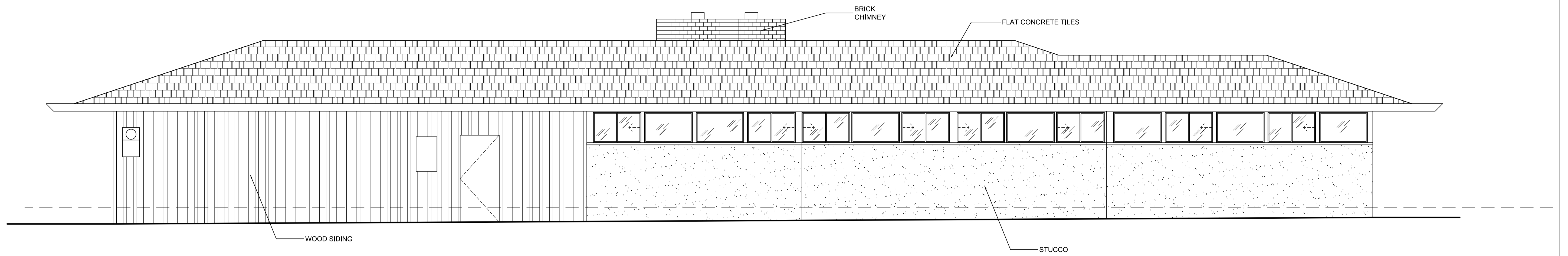
1 W. ELEVATION
